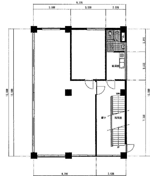
2F・3F平面図 専有面積97.58㎡(29.51坪)×2
