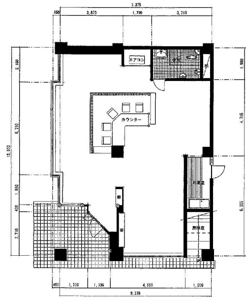
1F平面図 専有面積111.15㎡(33.62坪)
