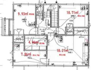
2階平面図
